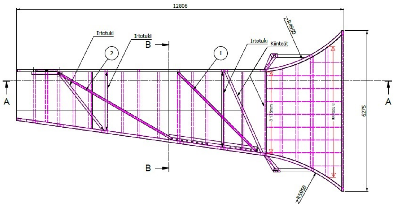
Kuva 2: Alasvaellusväylän suppilo ylhäältä kuvattuna. Vedenalainen kuvaus toteutetaan suppilon kohdassa, jossa leveys on vähän yli 3 metriä. Keskelle asennetaan pitkittäissuunnassa ohut muovilevy.
