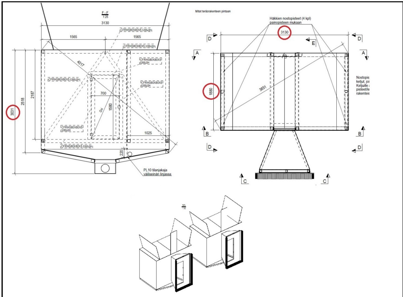
Kuva 3: Kiinniottohäkit. Punaisilla ympyröillä on merkattu häkkien mittoja: leveys 3130 mm, syvyys 1880 mm ja korkeus kaukalon kanssa 3031 mm.
